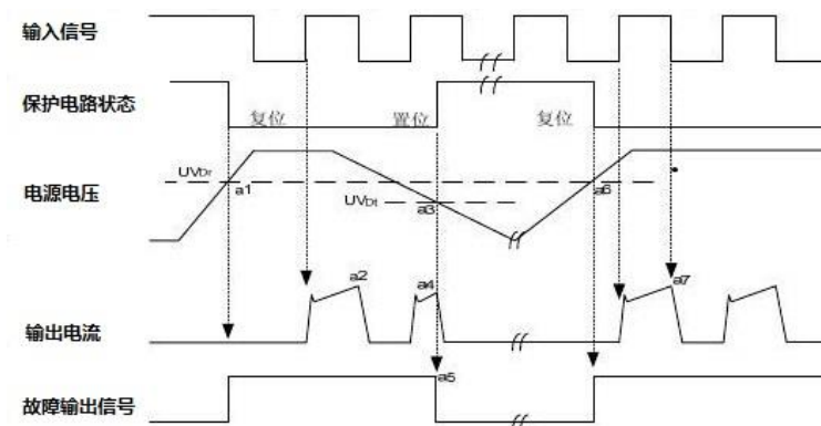
图 12: 欠压保护时序图(低侧)
