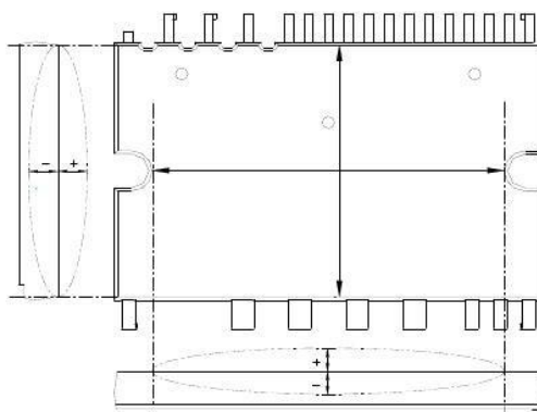
图 9: 平面度检测位置
